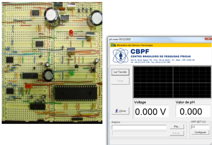
Protótipo de um Medidor de pH com correção de temperatura
