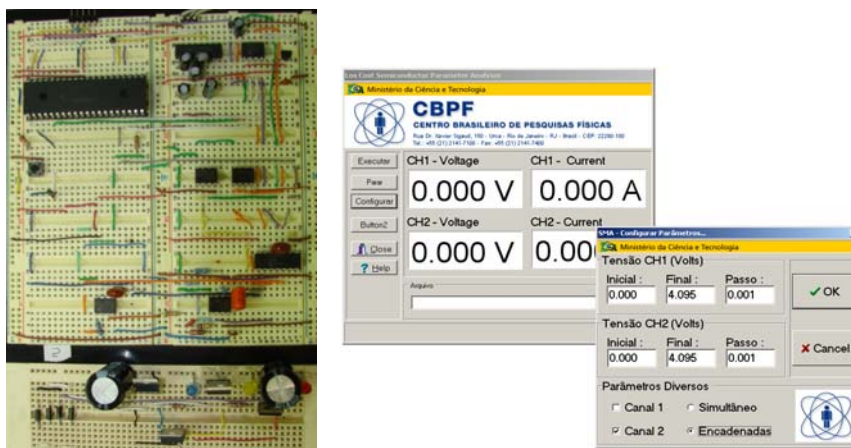
Protótipo de um analisador de parâmetros para caracterização elétrica do EGFET como sensor de pH em modo D.C
